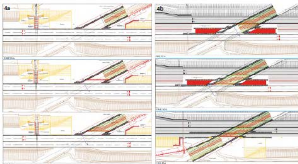
Figg. 4a e 4b - Fasi di varo
